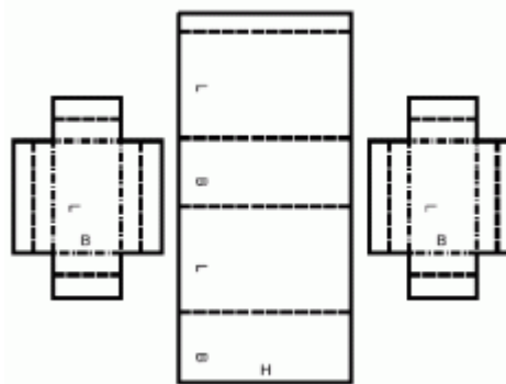
FEFCO 0615 M/A
