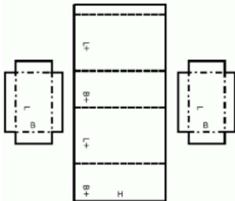
FEFCO 0616 M/A
