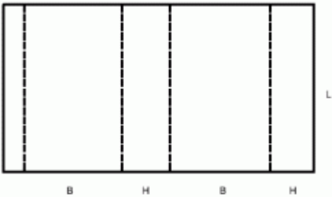
FEFCO 0503 M
